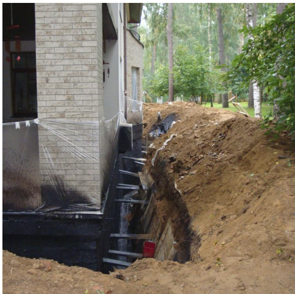
27-09-FL. Ремонт гидроизоляции фундамента
