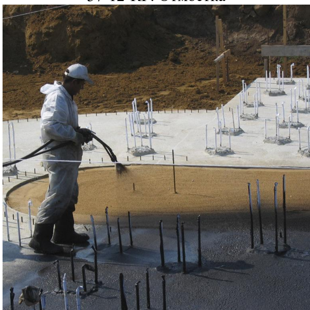
12-07-FL. Плавающая фундаментная плита
